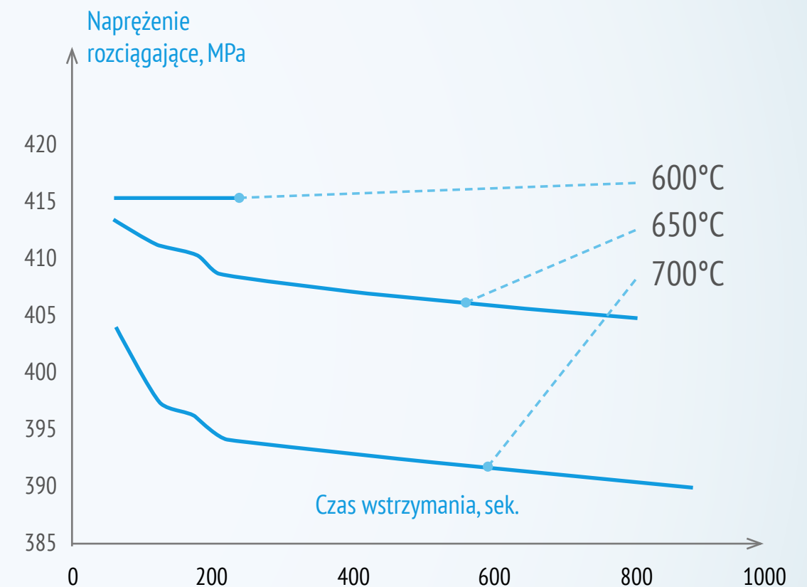
Mechaniczne właściwości mosiądzu na rury
